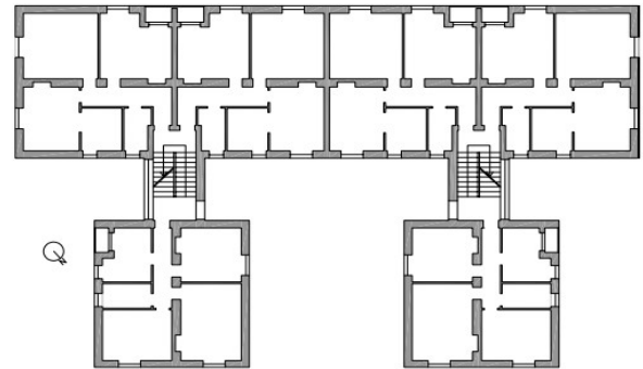
pianta piano tipo
